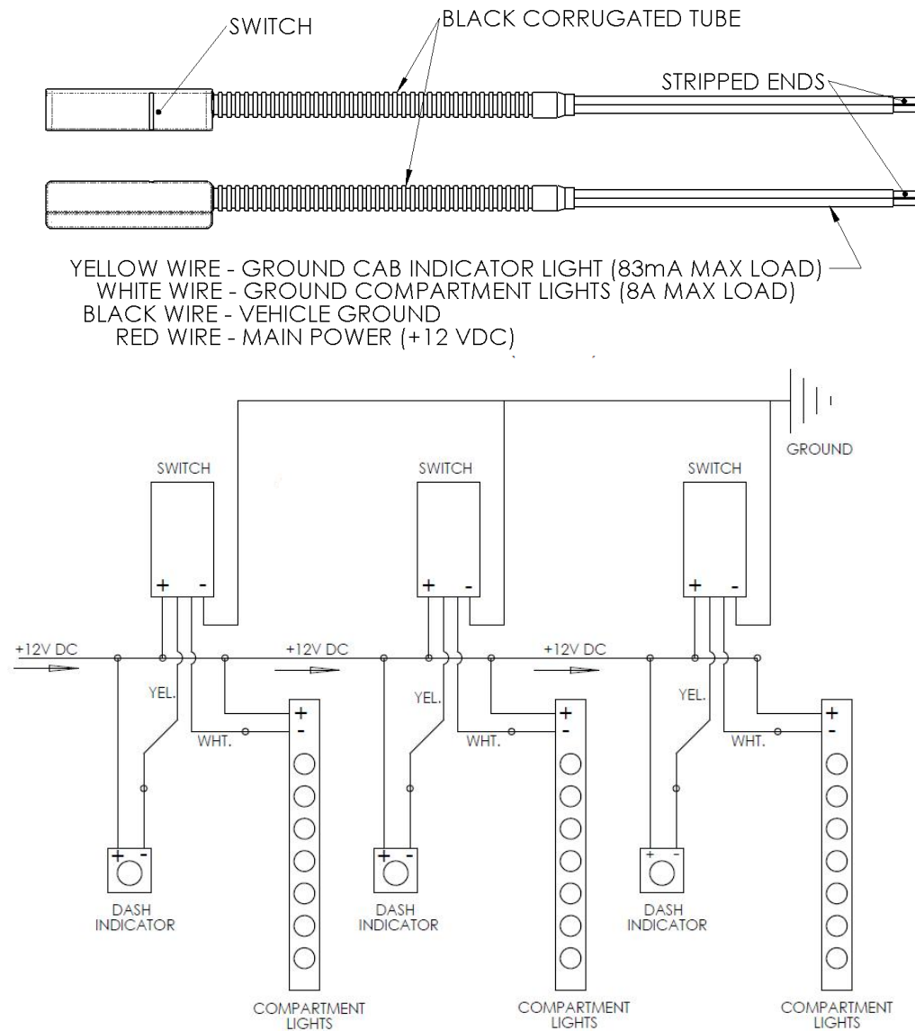
Fig. 19– Door ajar switch wiring
